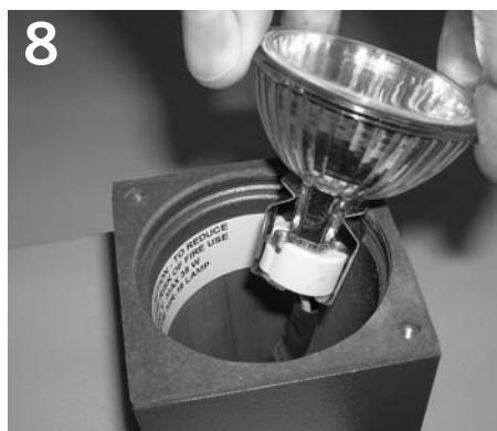
8 Install lamps per relamp label.
