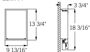
ZENN T4
