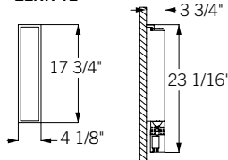
ZENN T2
