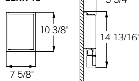
ZENN T3
