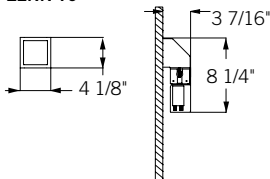
ZENN T0
